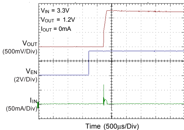
Soft-Start Function
