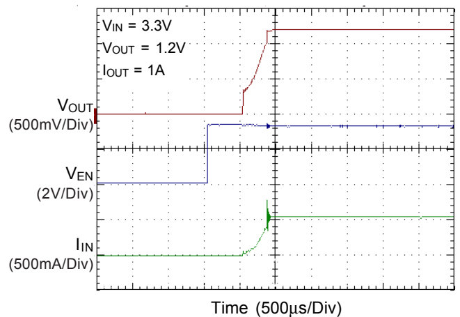
Soft-Start Function
