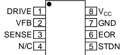
ZXSC440 (MSOP-8)
